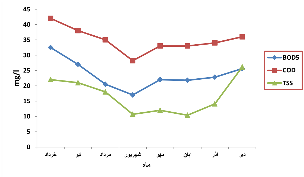
شکل ۲. تغییرات ماهانه غلظت پارامترهای BOD 5 , COD و TSS پس از خروجی از تصفیه‌خانه فاضلاب مهدی‌شهر در دوره تحقیق
